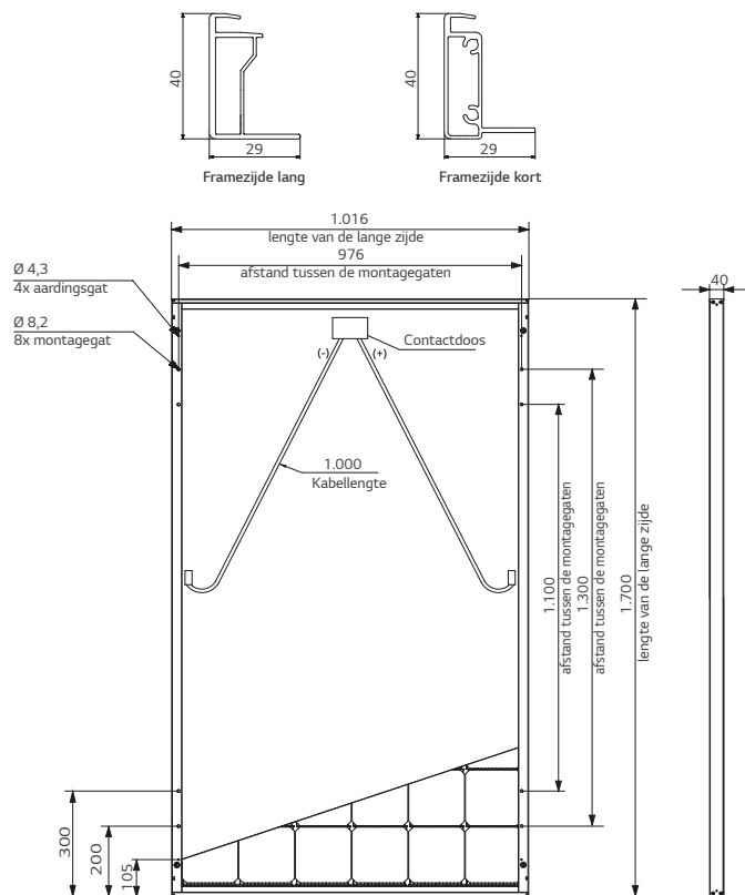
De afstand geldt tussen de middelpunten van de montage- en aardingsgaten.
